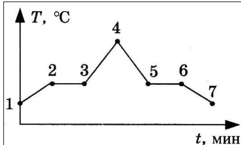
Рис. 1. График кипения эфира
